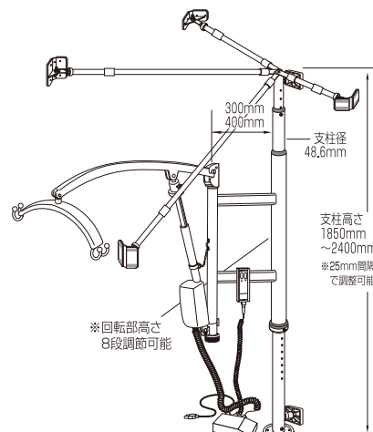
■F2RSKKセット外観寸法
